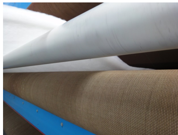
Bild 4: Die schrumpffresistenten Trocknerbänder von GKD gewährleisten eine ebenso kostensparende wie umweltschonende Klärschlamm-trocknung.
