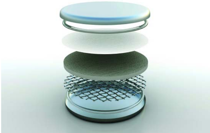
Bild 5: Spezialgewebekonstruktionen von GKD finden als Komponenten für alternative Antriebstechnologien wie Batterien oder Brennstoffzellen Einsatz.
