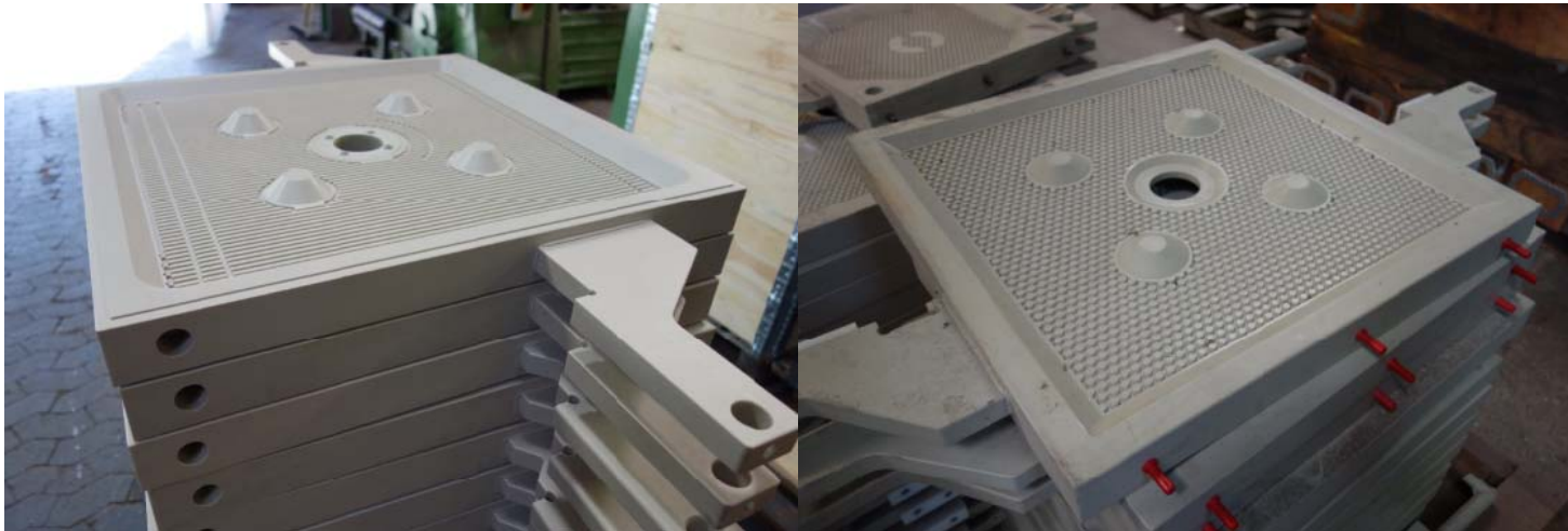
Bild 9-10: Das Filtrat fließt bei den Kammerfilterpressen über rillen- oder noppenrörmige Ablaufkanäle der Platten ab.
